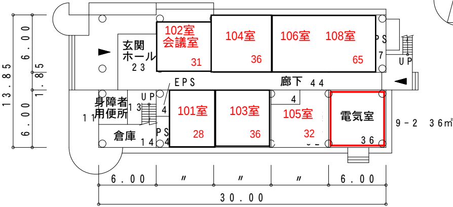
1階平面図 388㎡
