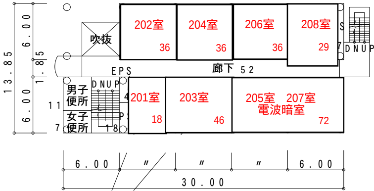
2階平面図 376㎡
