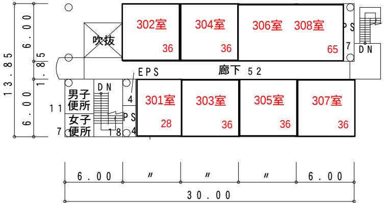
3階平面図 376㎡
